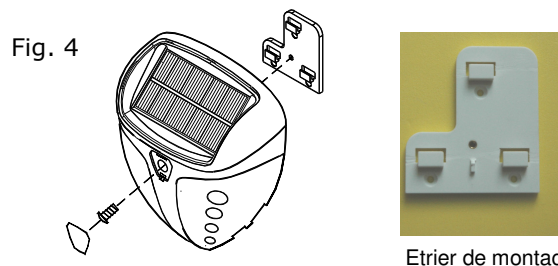
Etrier de montage
